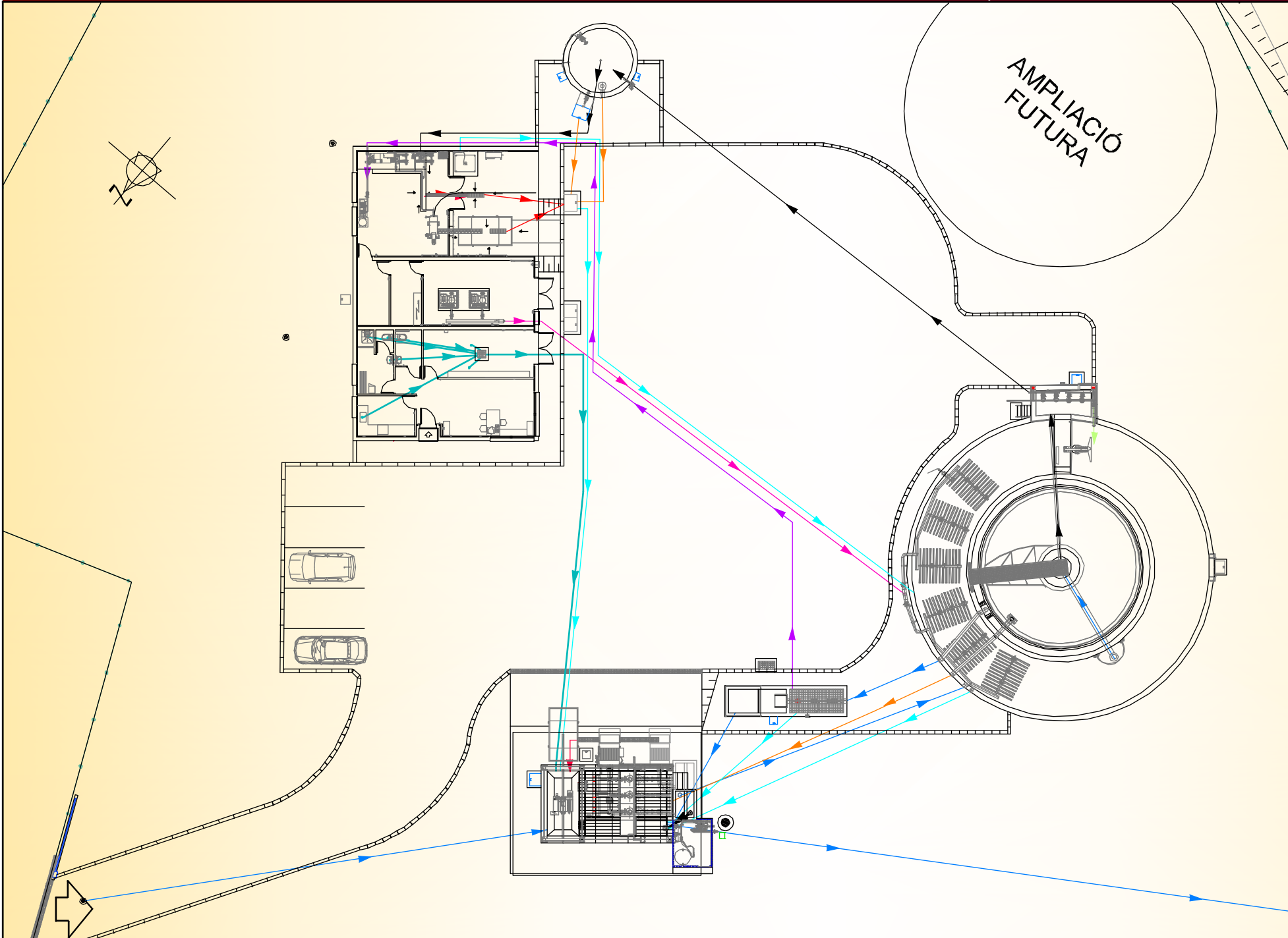
COL·LECTOR D'ARRIBADA, POU DE GRUIXOS I BY-PASS GENERAL DE LA PLANTA
