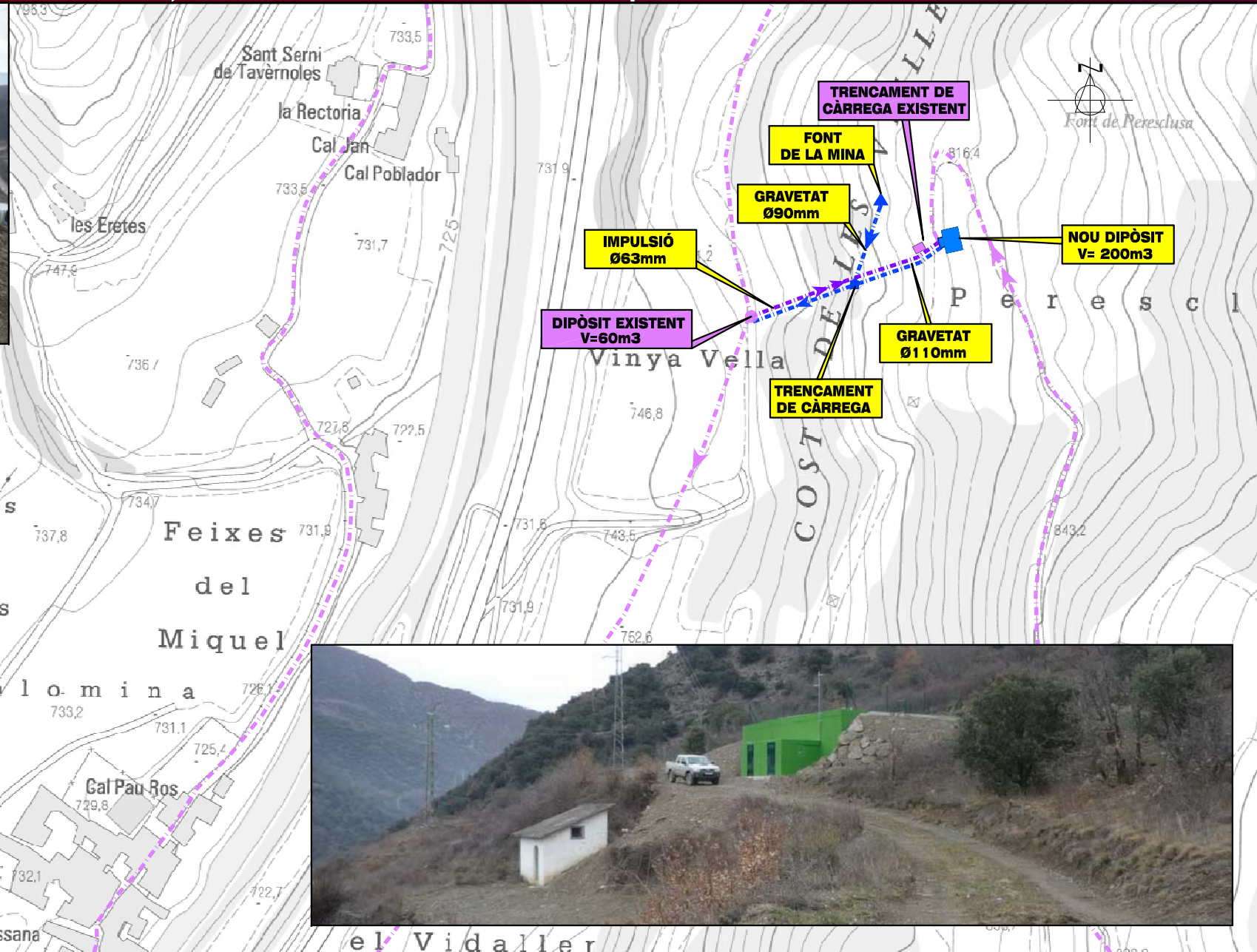
ESQUEMA XARXA NUCLI D'ANSERALL
