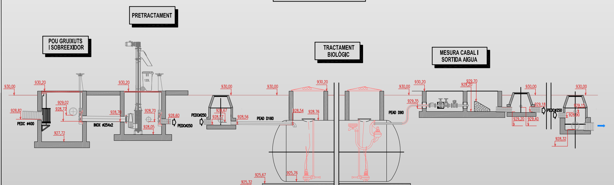
PERFIL HIDRÀULIC
