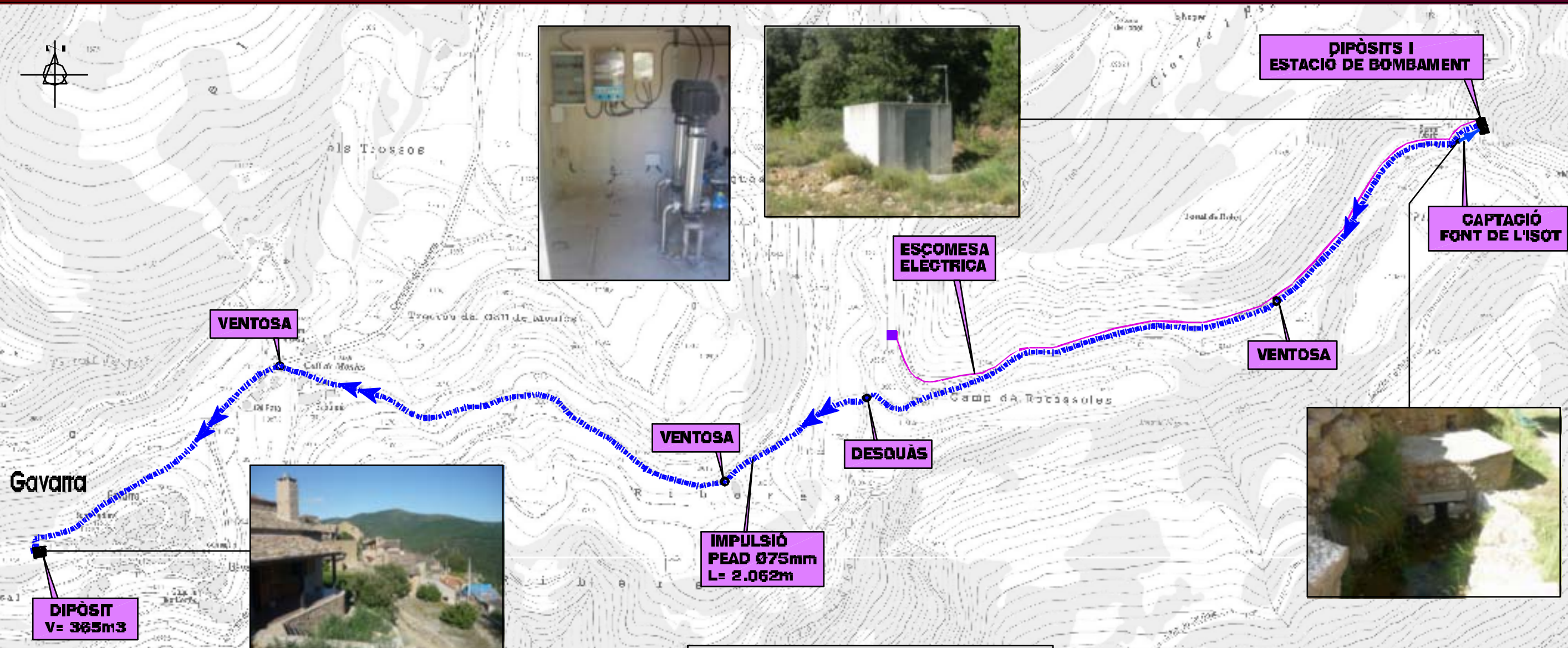
ESQUEMA DE LA XARXA DEL NUCLI DE GAVARRÀ
